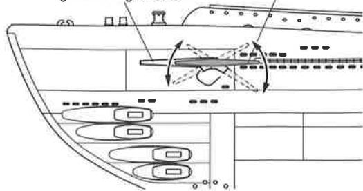
潜舵レセス Front diving rudder recess Nische der Tiefenruder Logement des gouvernes avant
