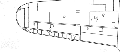
●52型の主翼 32型の翼端を半円形に整形。運動性を高めた。
