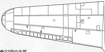
●32型の主翼 21型の主翼先端を50cm切りつめ、軽量化と速度の向上を図った。
