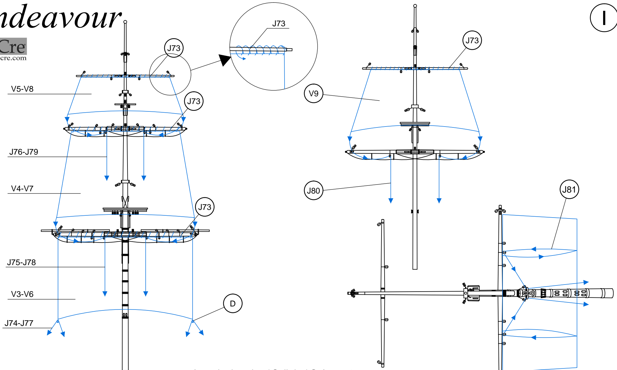
Aparejo de velas / Sail rig / Gréement Segel takelage / Sartiamе da vela
