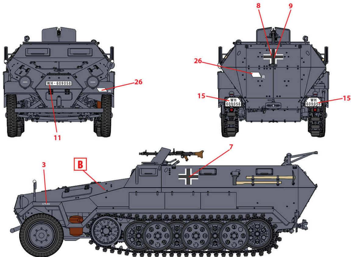
2. Sd.Kfz. 251/1 Ausf.A, 2.Pz.D., Греція, травень 1941 р. Sd.Kfz. 251/1 Ausf.A, 2.Pz.D., Greece, May 1941
