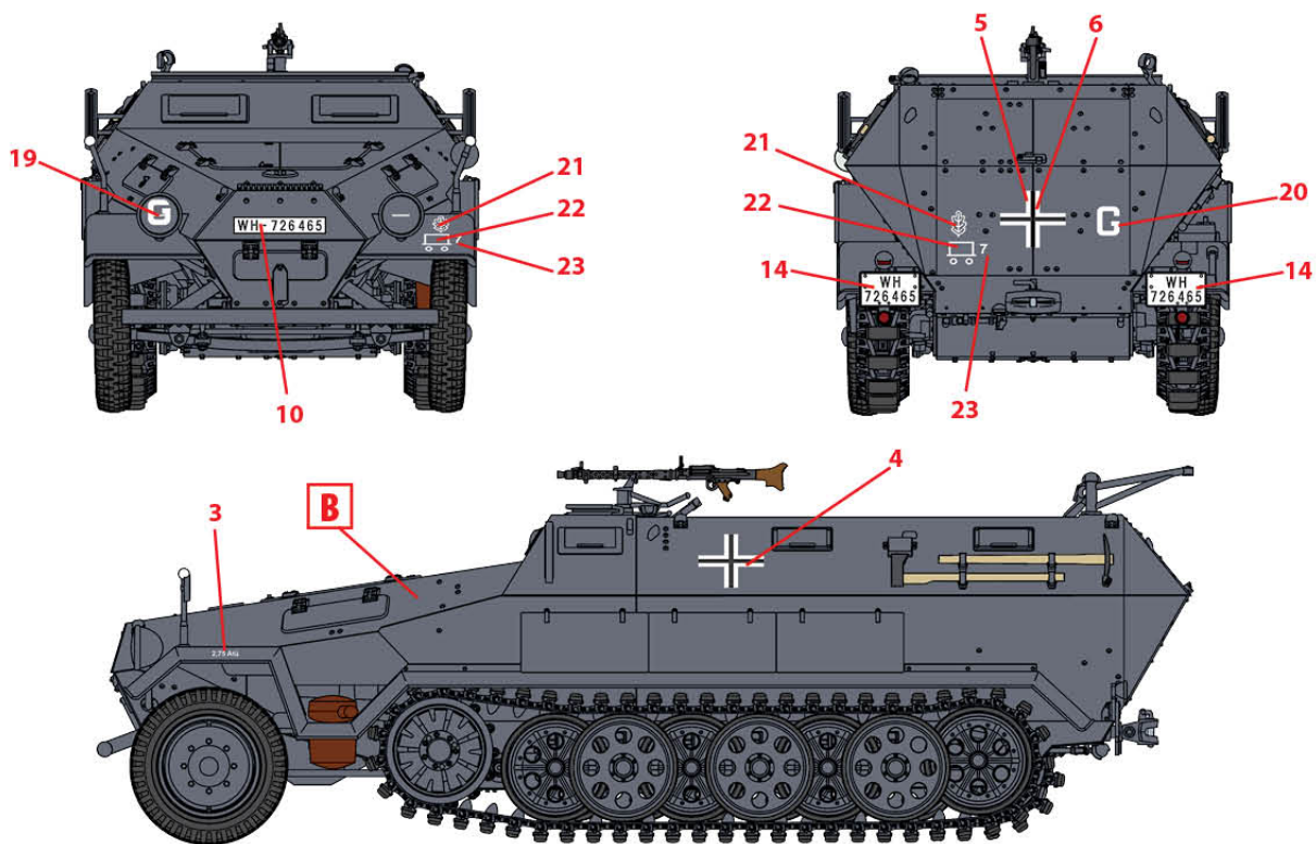
1. Sd.Kfz. 251/1 Ausf.A, 1.Pz.D., Франція, травень 1940 р. Sd.Kfz. 251/1 Ausf.A, 1.Pz.D., France, May 1940
