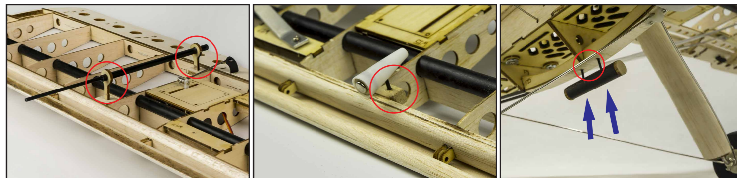
水平尾翼连接舵机 Horizontal tail connecting servo
